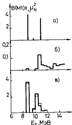
Рис.1. Вероятность электромагнитного возбуждения 1^+ -состояний в ядре ^{90}\text{Zr} : а) однофоновых состояний, б) двухфоновых состояний, в) состояний, описываемых волновой функцией (1) (пунктирная прямая - в выражении (2) учтен только член \sim R ; сплошная прямая - учтены оба члена в (2)).
