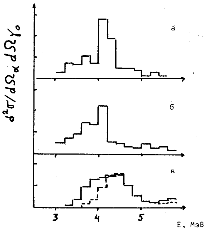
Рис.4. Сечения d^2\sigma/d\Omega_\alpha d\Omega_\gamma для реакции ^{112}\text{Sn}({}^3\text{He}, \alpha\gamma_0) /произвольные единицы/: а/ экспериментальные данные /15/, б/ экспериментальные данные /16/, в/ расчеты КФМ /28/.
